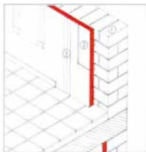
Isolamento verticale dall'interno
