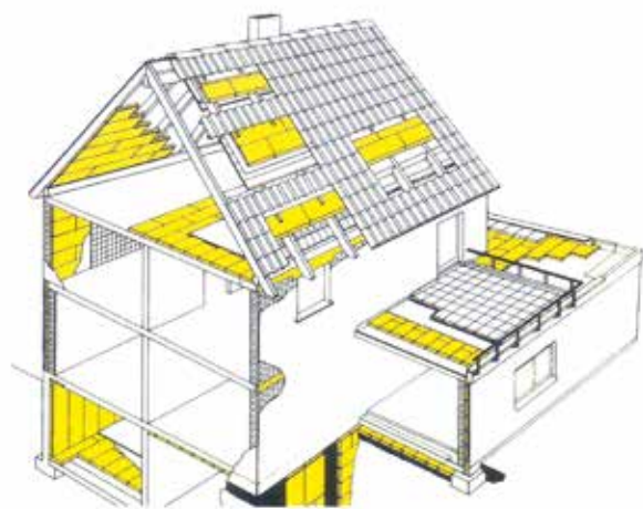
Esempi applicati dell'utilizzo del pannello in polistirene
